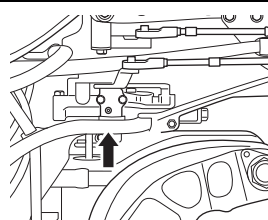
Dźwignia sprzęgła
